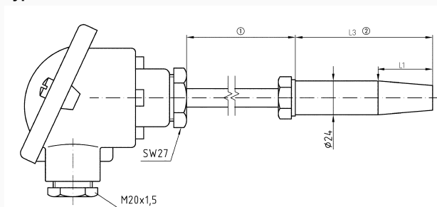
Typ WTh 26
