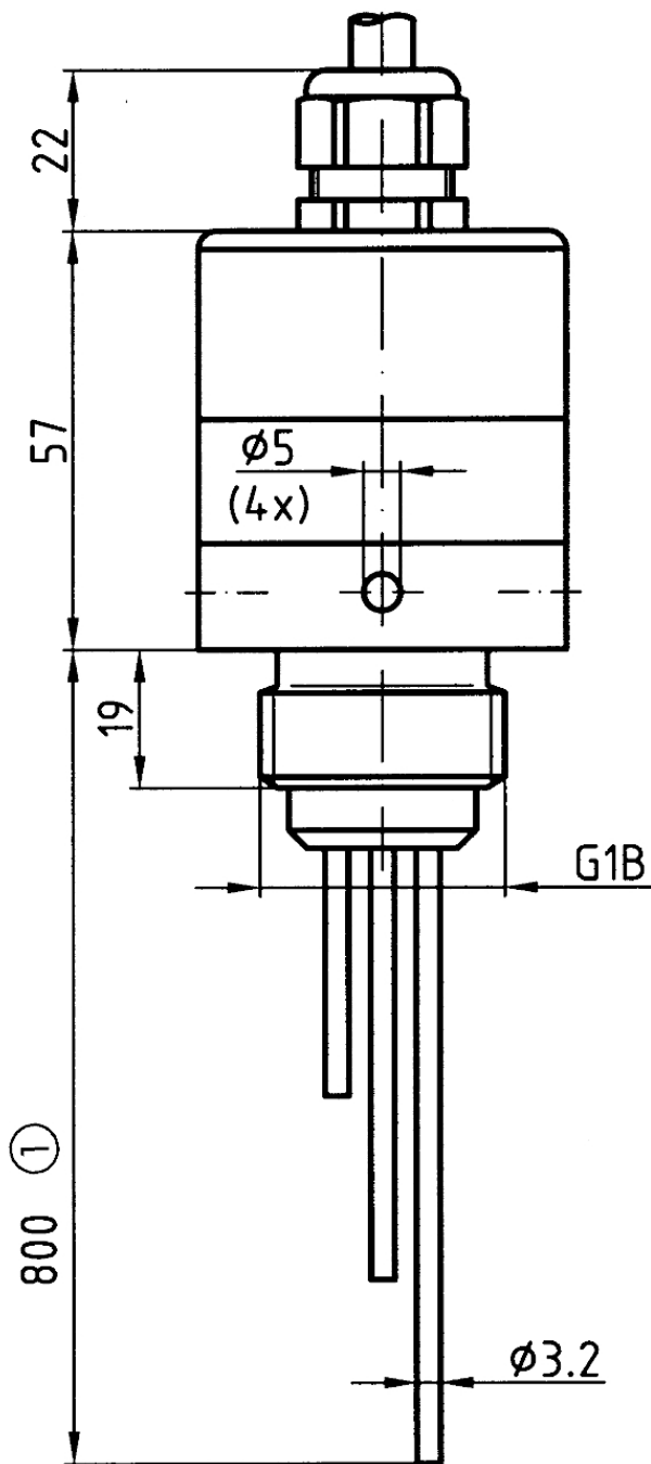
Dreistabsonde LSM 02
