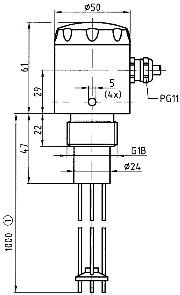
Dreistabsonde LSM 01
