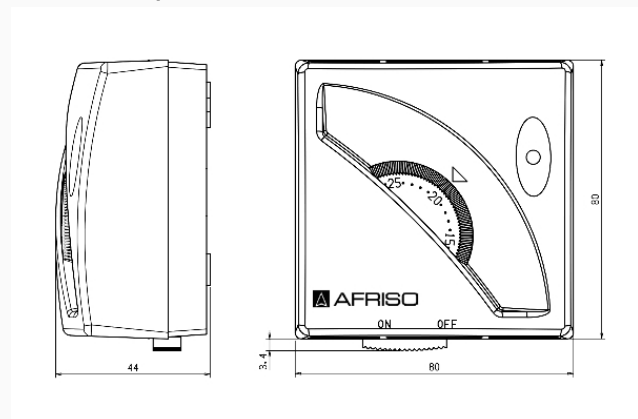
Masse (mm)
