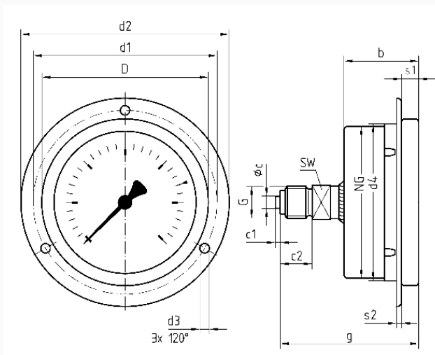
NG 63 – Anschluss axial exzentrisch, 3-Lochfrontflansch
