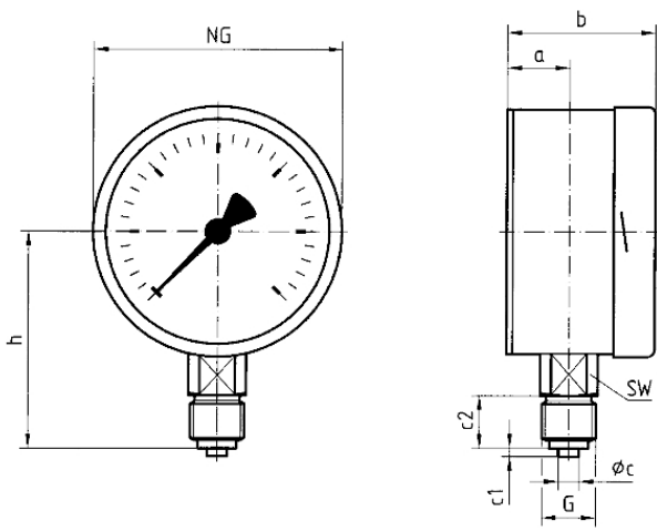
Masse (mm)
