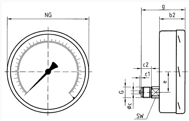
Maße (mm)
