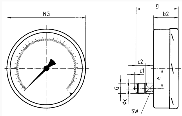
Maße (mm)
