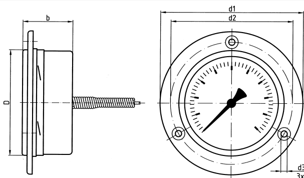
Ausführung mit Fernleitung und 3-Lochfrontflansch
