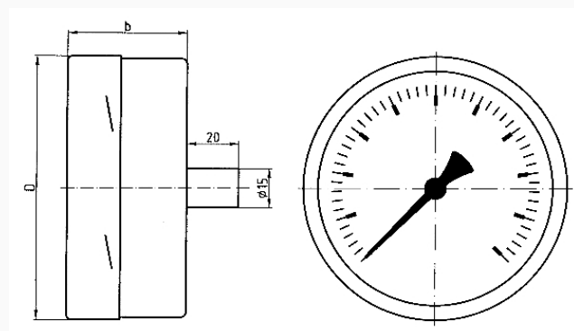
Anschluss axial
