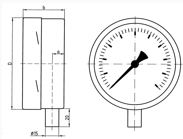
Maße (mm)
