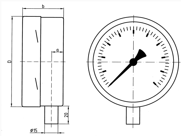
Maße (mm)
