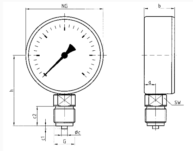
Masse (mm)
