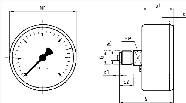
NG 40/50/63 – Anschluss axial
