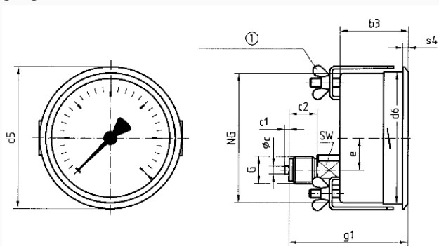
Anschluss axial, exzentrisch, 3-Kantfrontring mit Bügelbefestigung
