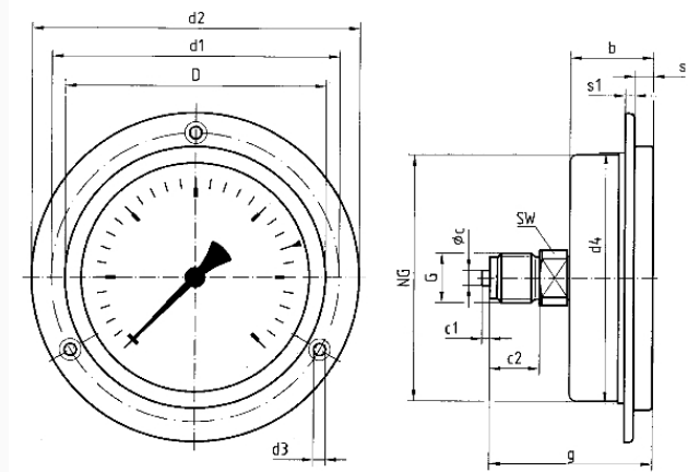
NG 100 – Anschluss axial, 3-Lochfrontflansch
