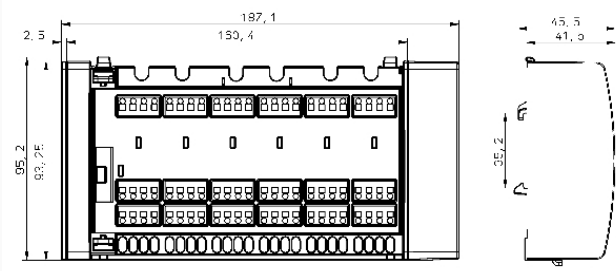
CosiTherm® Basic Klemmleiste WB 10-D 8-230
