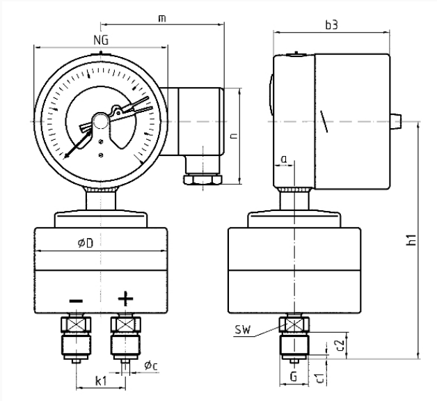
Masse (mm)
