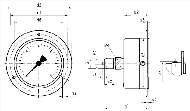
Anschluss axial, 3-Lochfrontflansch
