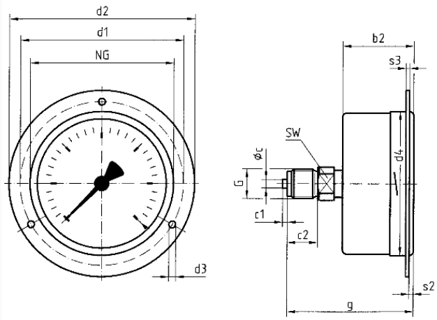
Masse (mm)
