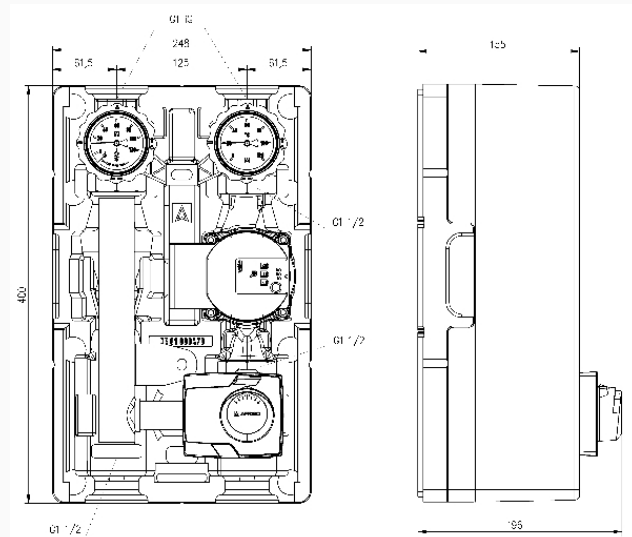
PrimoTherm® 180-2 mit Wilo-Pumpe
