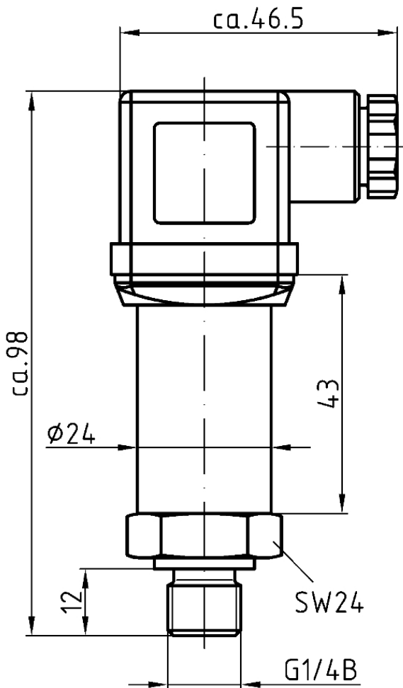
DMU 01 K - Anschluss G \frac{1}{4} B EN 837
