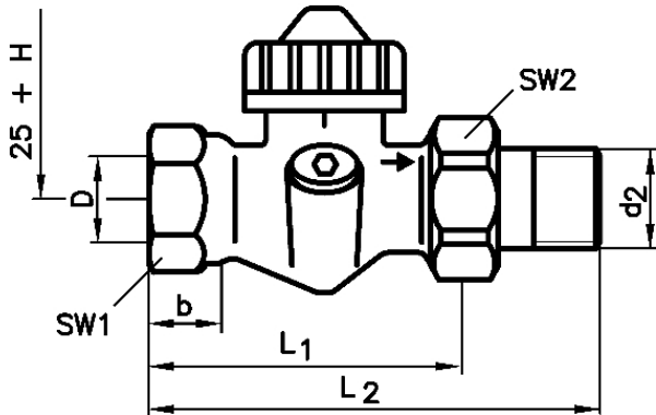
Bauformen und Masse gemäss EN 215, Baureihe D
