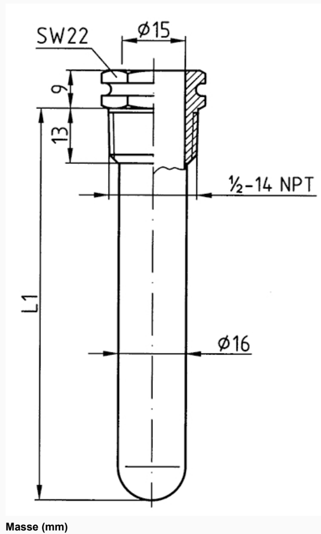
Tauchhülse ½" 15 x 16 mm
