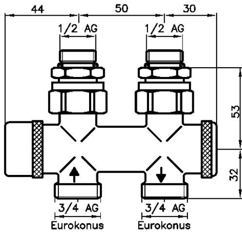
456-DP, Durchgang – Ausführung G \frac{1}{2} -Aussengewinde
