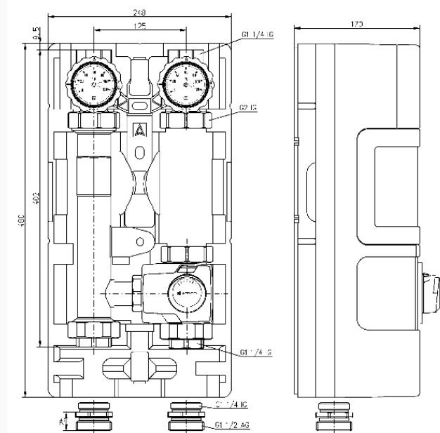
PrimoTherm® K 180-2 DN 32 KSV Vario
