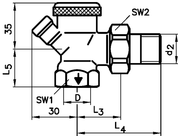
Bauformen und Masse (mm) gemäss DIN 3842
