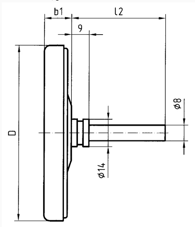
Anschluss axial, glatt
