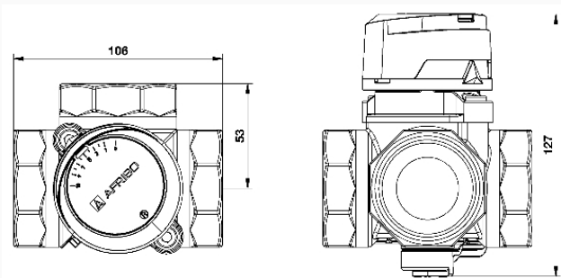
3-Wege-Mischventil DN 50
