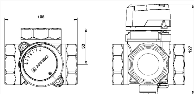
3-Wege-Mischventil DN 40
